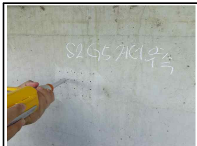
반발경도 시험
