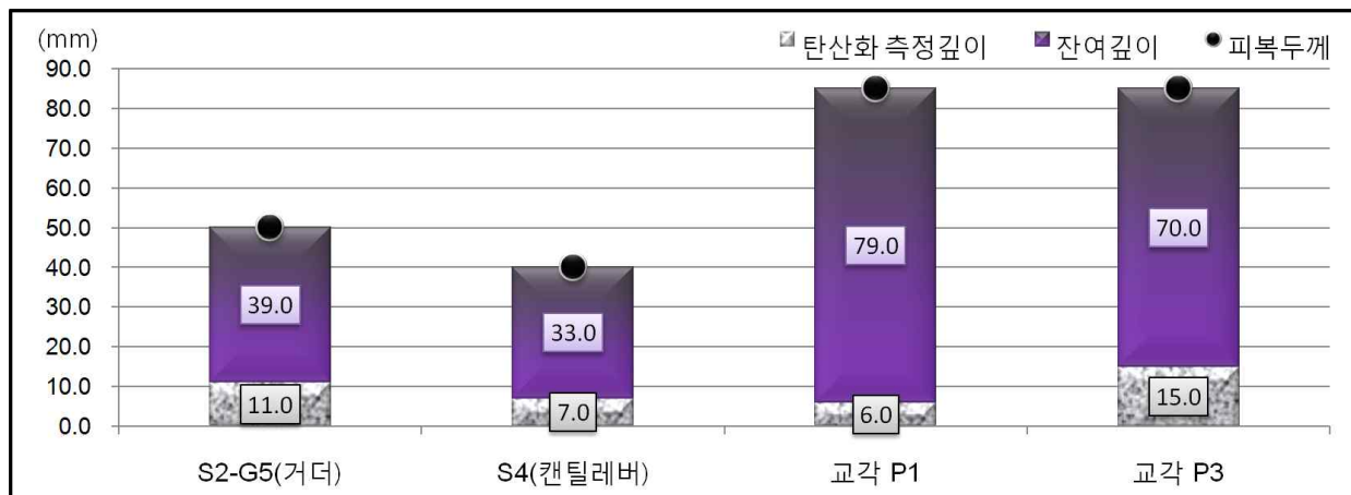
【그림 4.3】 탄산화 진행깊이 및 잔여깊이 측정결과
